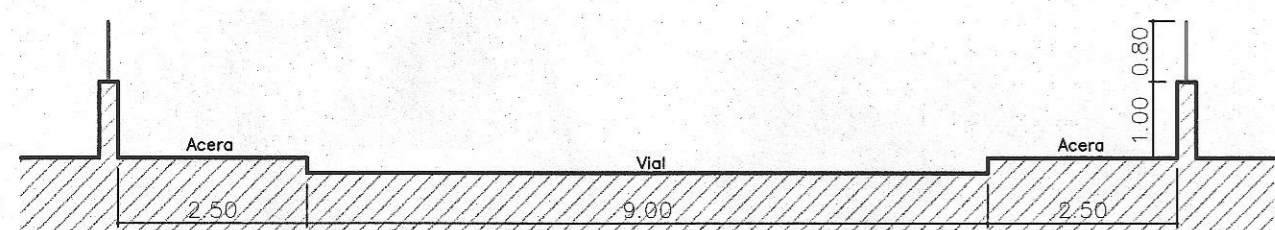
SECCIÓ 3-3 VIAL "K"
