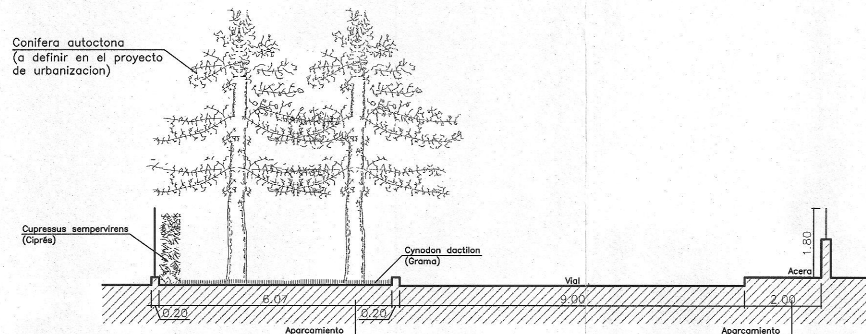
SECCIÓ 4-4 VIAL "K"
