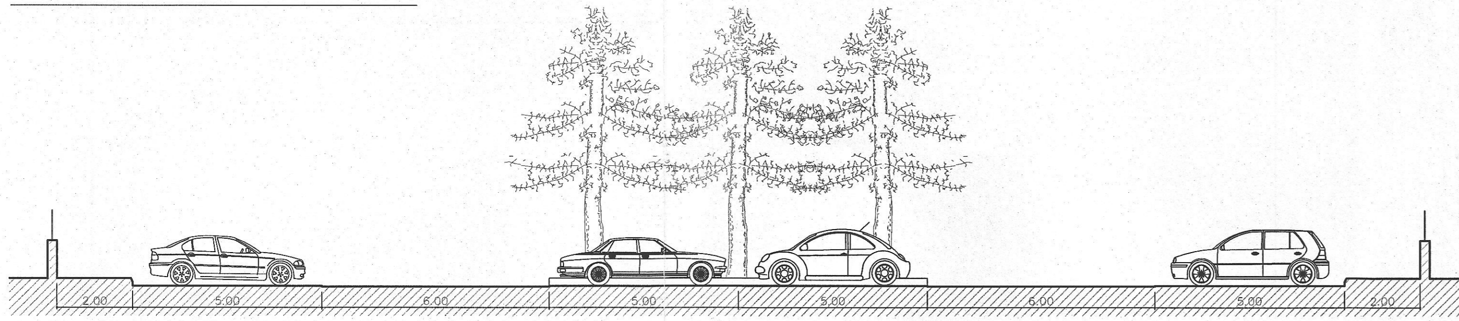
SECCIÓ 1-1 VIAL APARCAMENT
