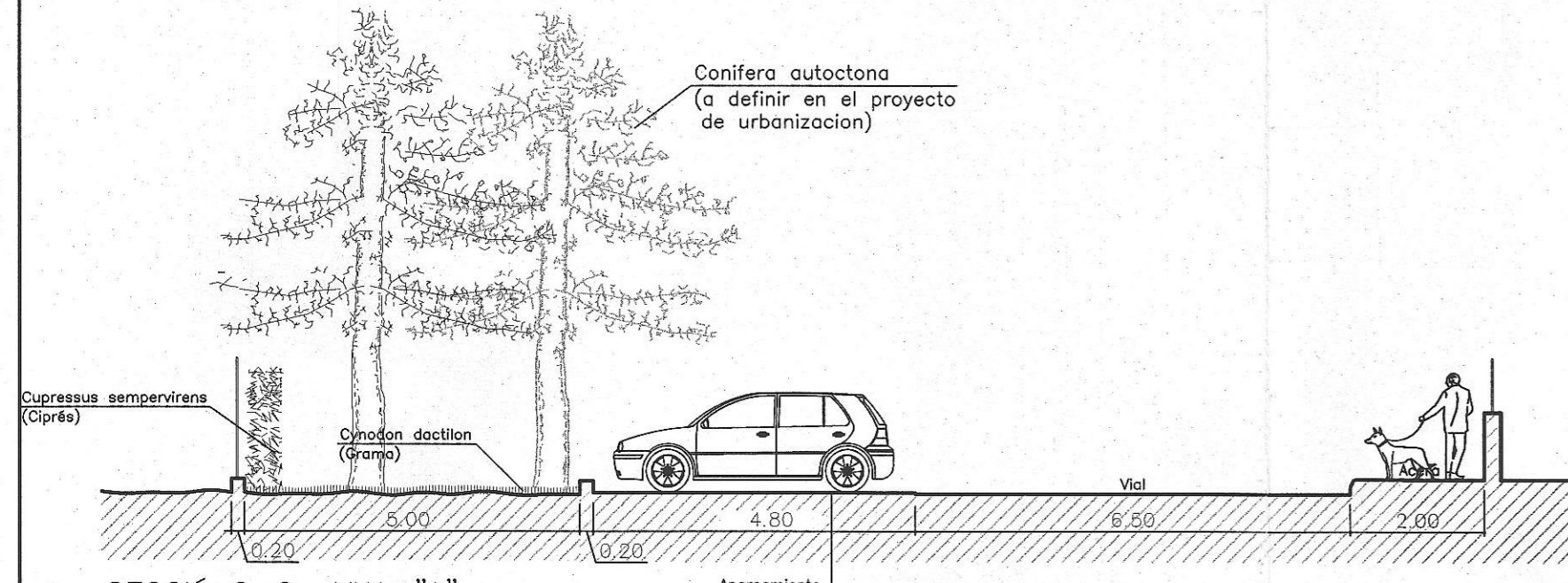
SECCIÓ 2-2 VIAL "A"
